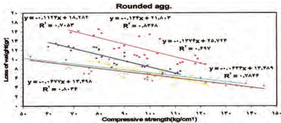
شکل ۹ - تغییرات نزولی مقدار کاهش وزن نمونه‌ها ناشی از فرسایش نسبت به مقاومت فشاری نمونه‌های رودخانه‌ای زمان (سن نمونه) و نوع دانه بندی دارد
