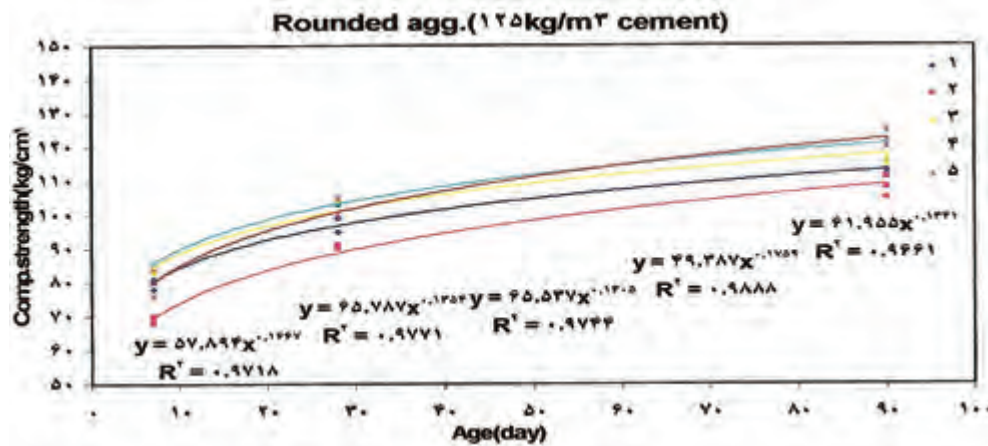
شکل ۷- منحنی تغییرات مقاومت فشاری نمونه های رودخانه ای نسبت به سن نمونه برای مقدار سیمان ۱۲۵ kg/m³
