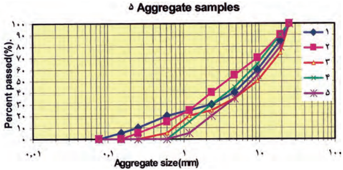
شکل ۴ - منحنی‌های پهن‌گانه دانه‌بندی
